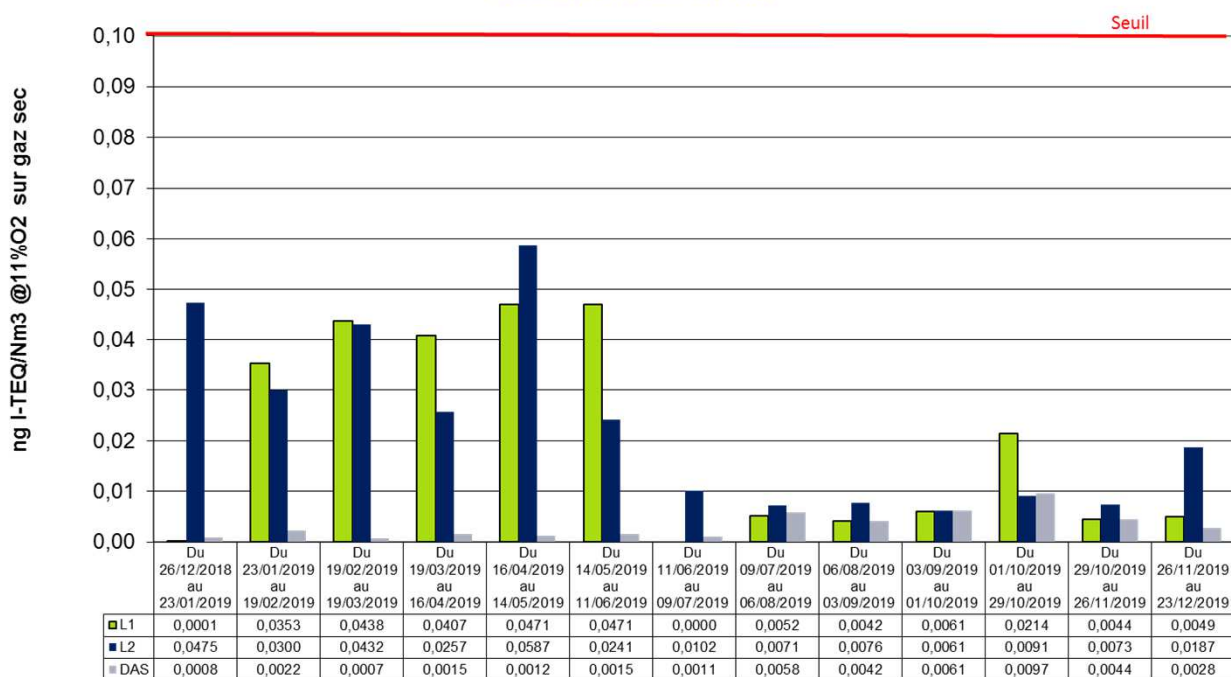
UVE VLM - Teneurs en PCDD/F en I-TEQ Mesures en semi-continu
